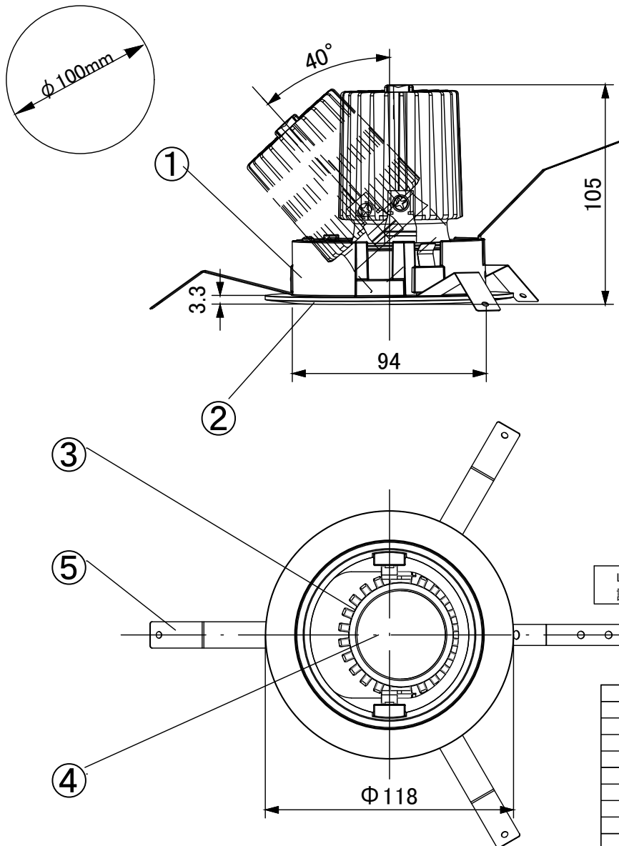
天井切込寸法
