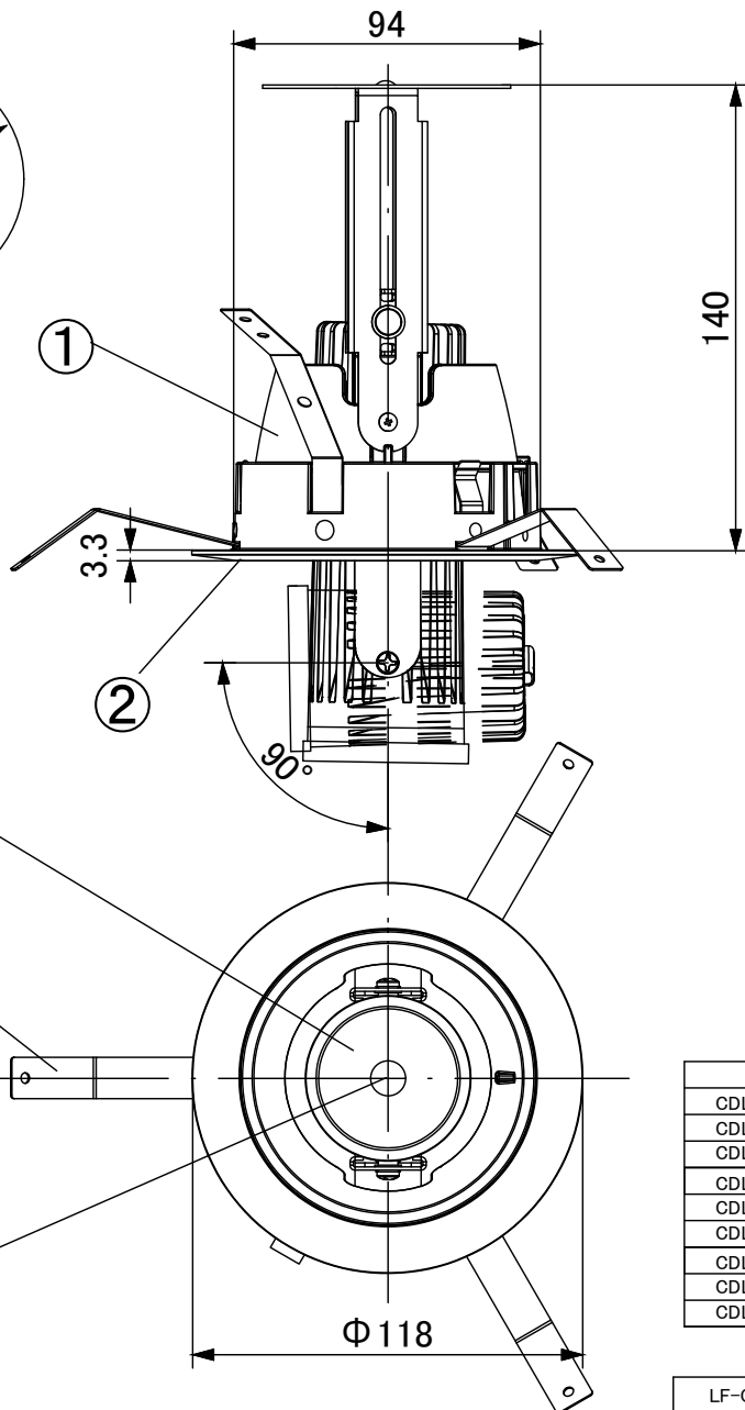
天井切込寸法
